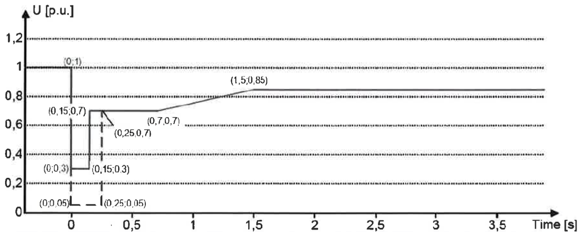
Figur 2 Synchron generatorteknologi skal kunne tåle underspenninger i henhold til den heltrukne linjen i denne figuren (skal tåle spenninger/tidspunkter som ligger over linjen)
